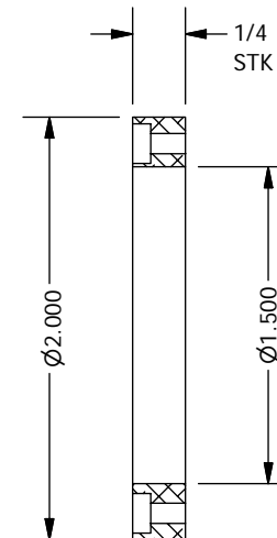
SECTION A-A SCALE 1 : 1
