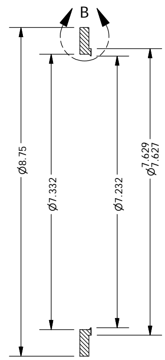
SECTION A-A SCALE 0.40 : 1
