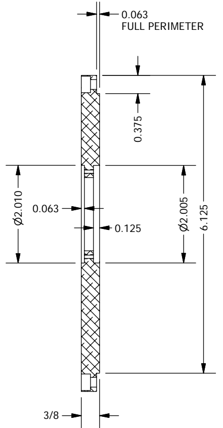
SECTION A-A
